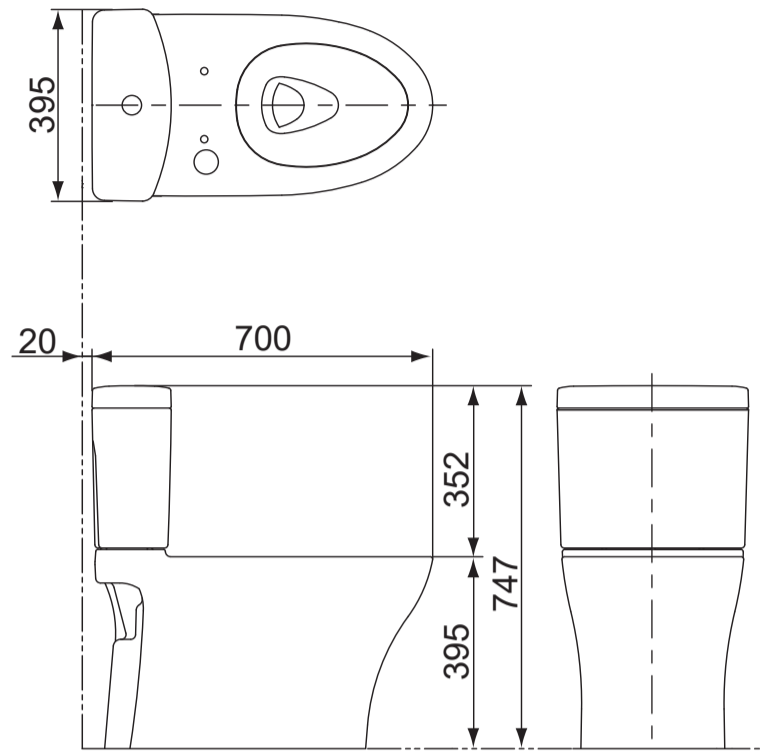
Sơ đồ lắp đặt sản phẩm CS769***
