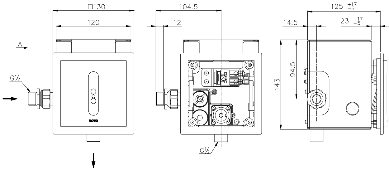
Nhìn t? A/ View A
